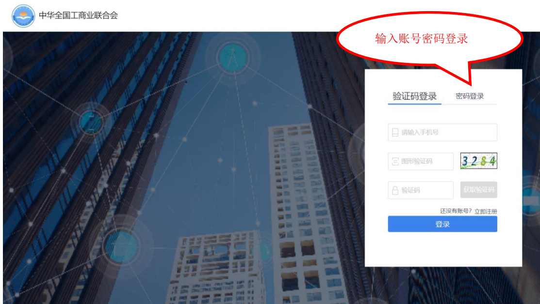
图 4 登录页面
